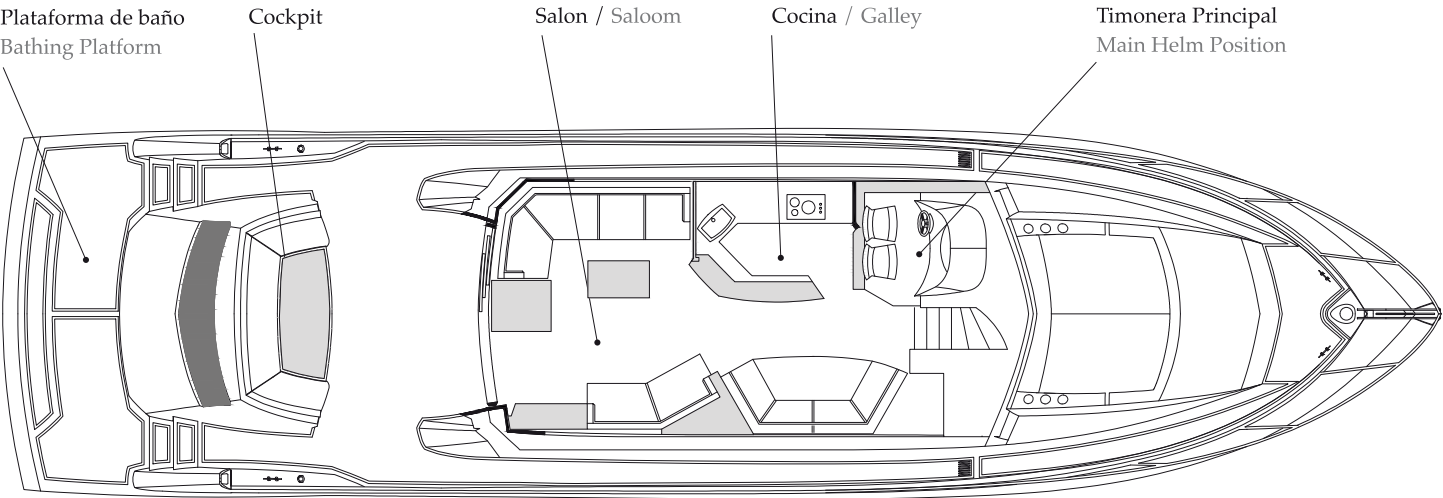
Planta de Cubierta / Upper Accomodation Layout
