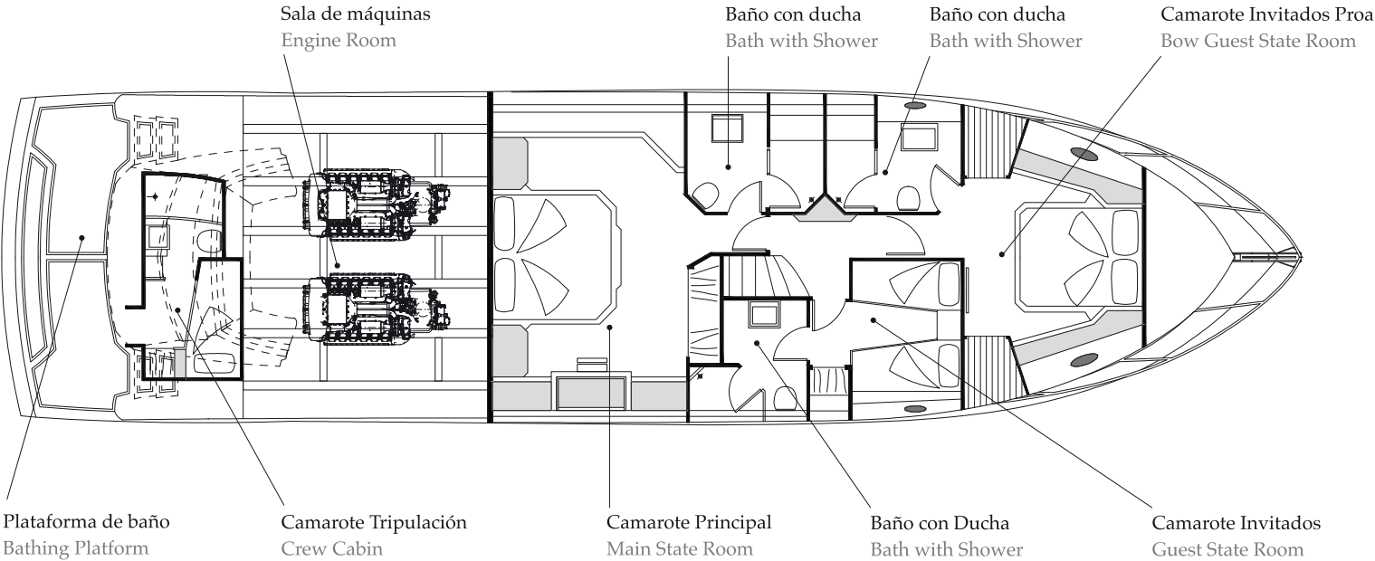
Planta de Interiores/ Lower Accomodation Layout
